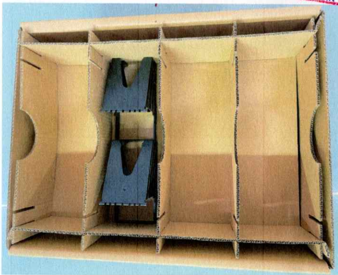
图二，将 PA4360 按照如图的方式放入内箱中，一箱 2 层，1 层 4 格，一格装两个产品，一箱共 16 个。
